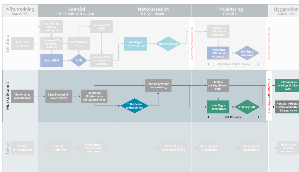
Figur 5. Arbetsströmmen Markåtkomst
