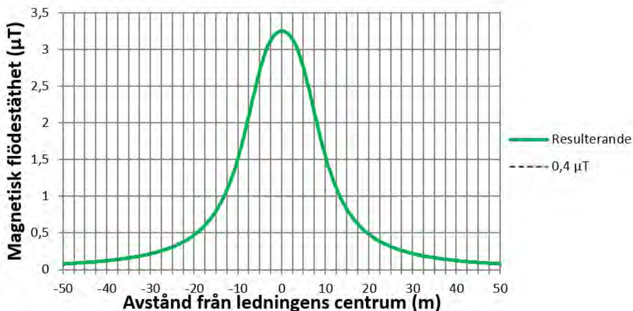
Figur 5-4. Beräknad magnetfältsnivå (grön kurva) för den nya ledningen Kopplingsstationen - Sandberget. 0 = ledningsgatans centrumlinje.
